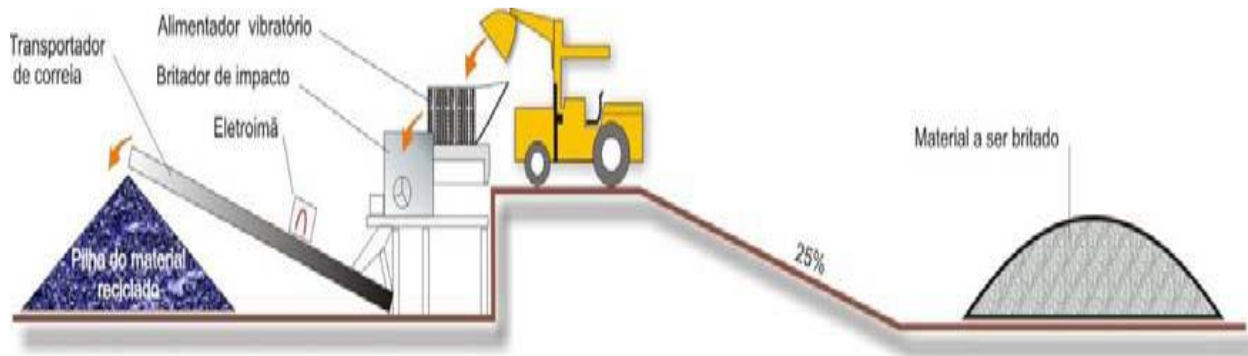
Figura: Representação Esquemática da Estação de reciclagem
