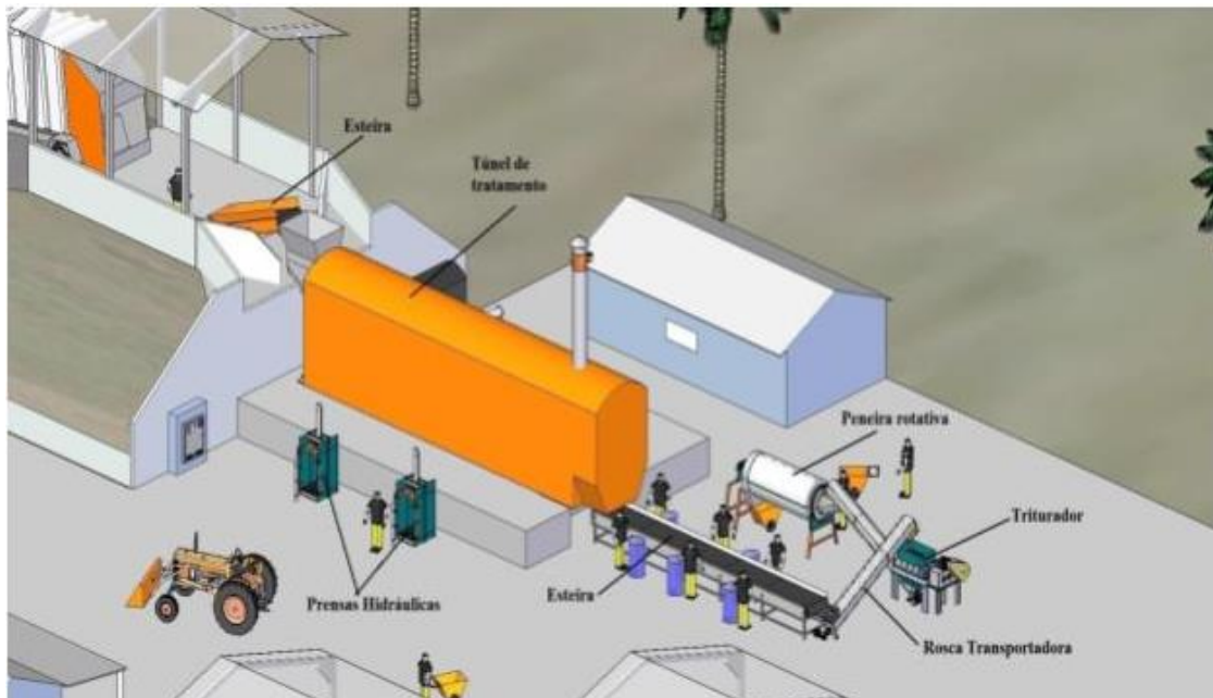
FIGURA 4: INFRA-ESTRUTURA DE UMA CENTRAL DE TRIAGEM E COMPOSTAGEM Fonte: UMUTORNO, 2015 (modificado).
